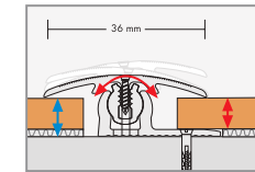
Übergangprofil Beidseitige Abdeckung durch Deckprofil: 12 mm/Seite
